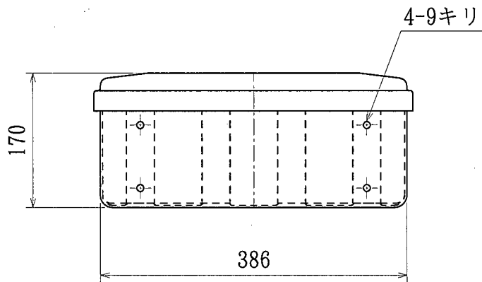
Z部詳細
